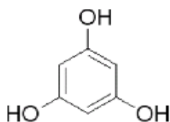
شکل 1: مولکول فلوروگلوکوسینول (1,3,5-Trihydroxybenzene)
